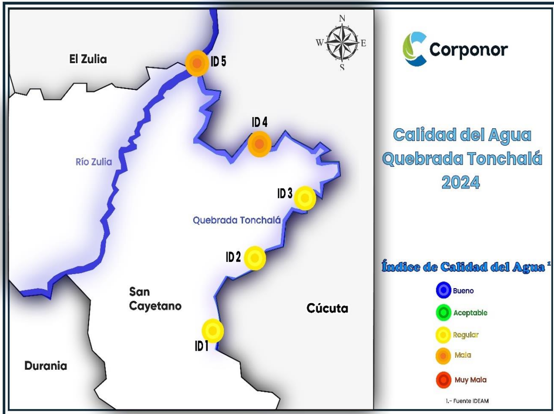
Figura 20. Mapa del comportamiento del ICA en la Quebrada Tonchalá.
